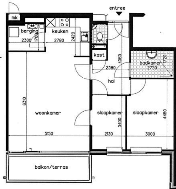
type C 3 kamer appartement
