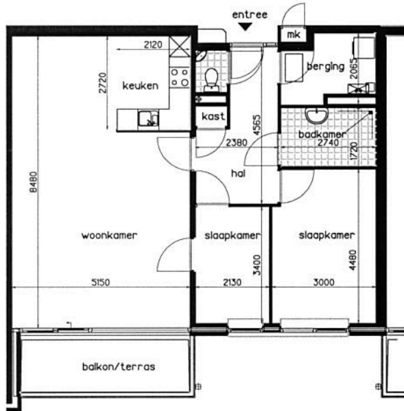
type B 3 kamer appartement
