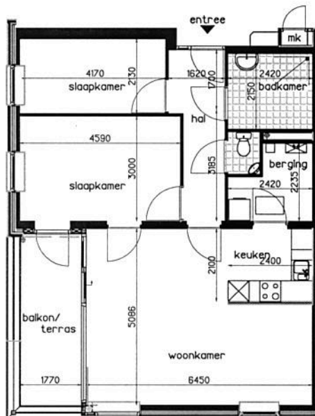
type D 3 kamer appartement
